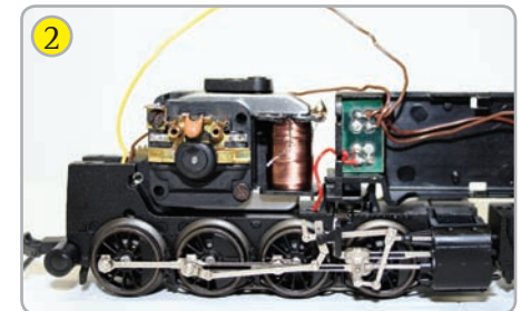
2 Allstrommotor mit angeschl. Delta-Decoder. Entfernen Sie alle Drähte zwischen Motor und Decoder und alle Entstördrosseln, außer dem zwischen den Motoranschlüssen.
