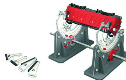
Wartungsbank 15.PLB-902 Mehrfach einstellbar rotierend
