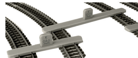
Parallelgleislehreset 15.PPT-H0-MK Für Märklin K-Gleis
