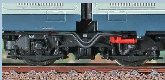
Dettaglio della riproduzione dei motori sui carrelli
